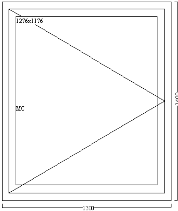
Чертеж изделия
