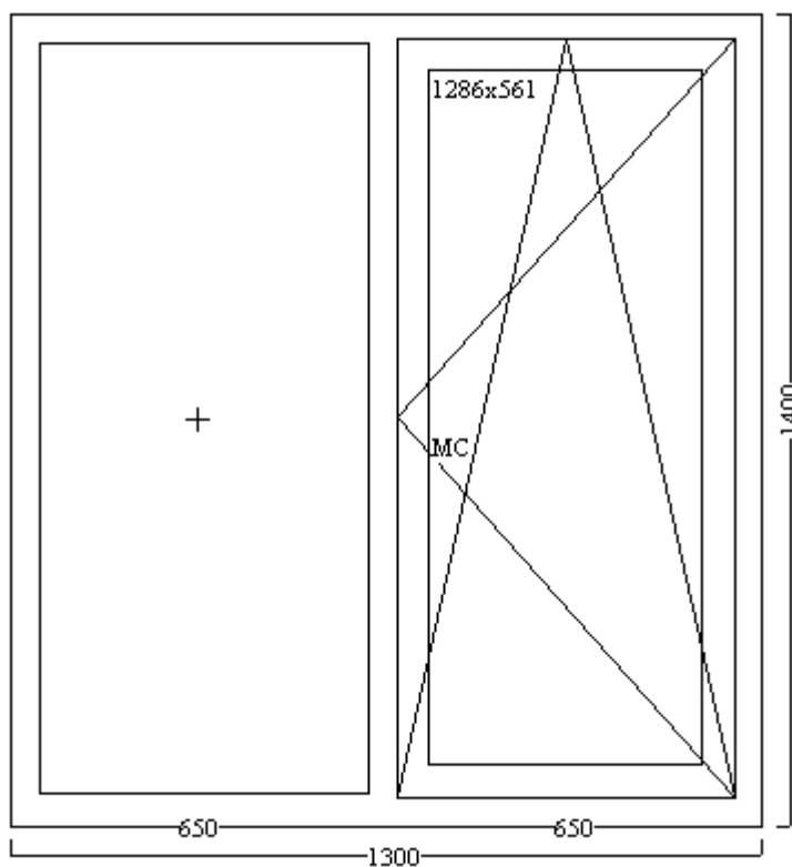
Чертеж изделия
